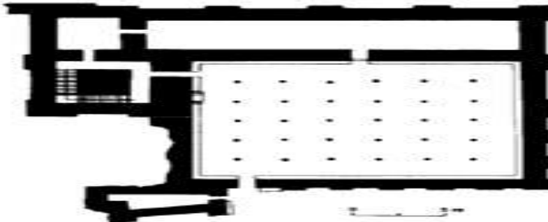
تصویر ۶- تالار ستوندار هخامنشی، اربونی (KNAUSS, 103)
